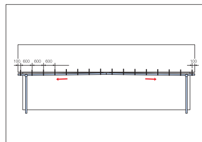
Две водосточные трубы на длине кровли, превышающей 10 м.
